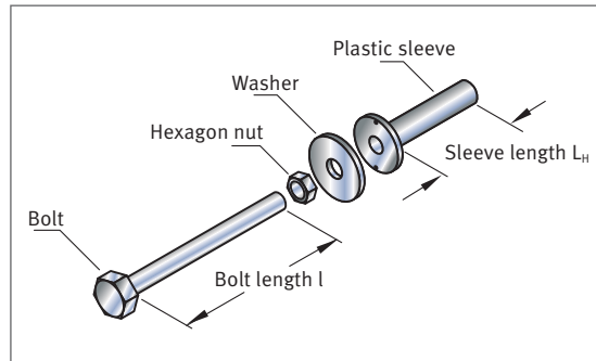
JORDAHL® Pressure bolt.
